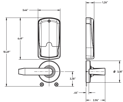
Mortise
